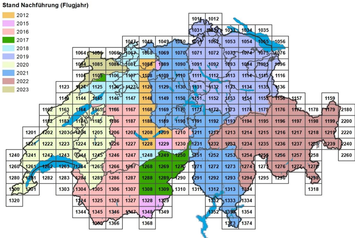
Abbildung 3: Nachführungsstand von swissALTI 3D -Ausgabe 2024, erste Edition
