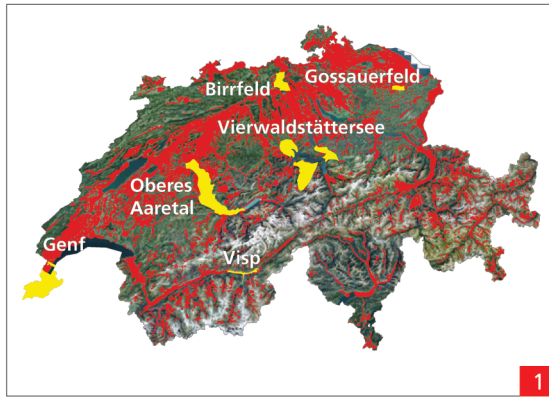
Fig. 1 Rot: bedeutende, an der Erdoberfläche kartierte Lockergesteinsvorkommen (gemäss Geologische Karte der Schweiz 1:500 000). Gelb: Perimeter der sechs GeoQuat-Pilotregionen.
