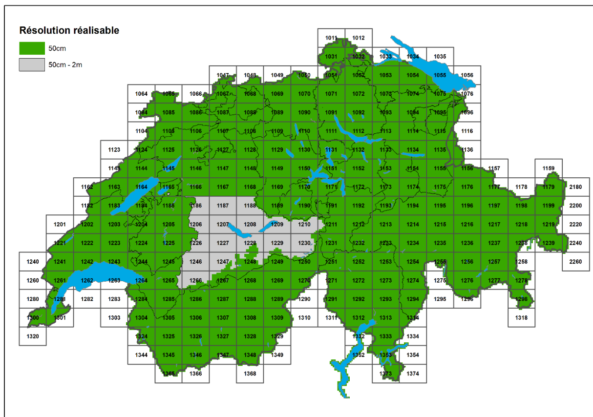
Figure 5: Résolution réalisable de swissALTI 3D en fonction de la densité de points des données de base
