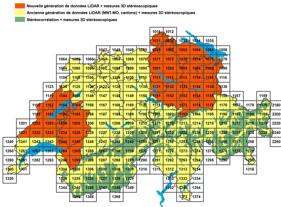
Figure 4: Méthodes de production utilisées pour l'élaboration de swissALTI 3D
