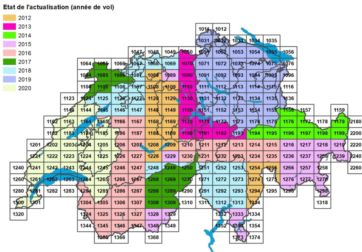
Figure 3: Etat de mis à jour de swissALTI 3D Version 2021, premier release
