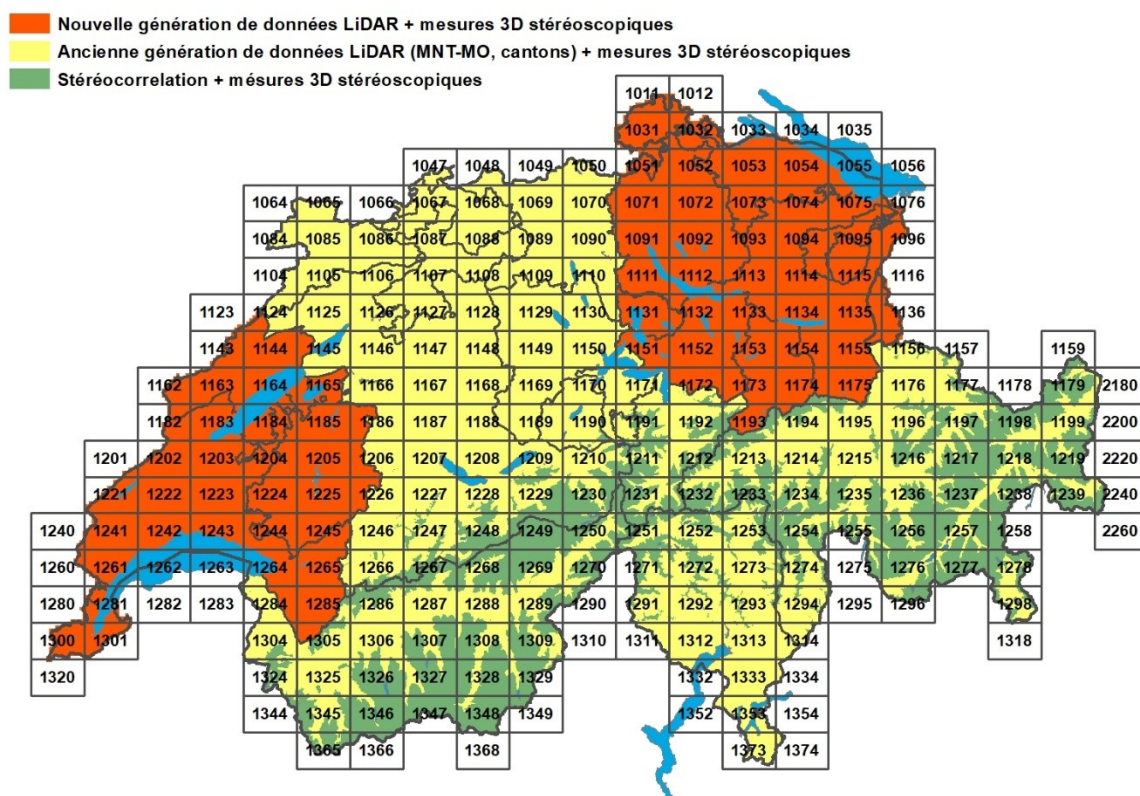
Figure 4: Méthodes de production utilisées pour l'élaboration de swissALTI 3D
