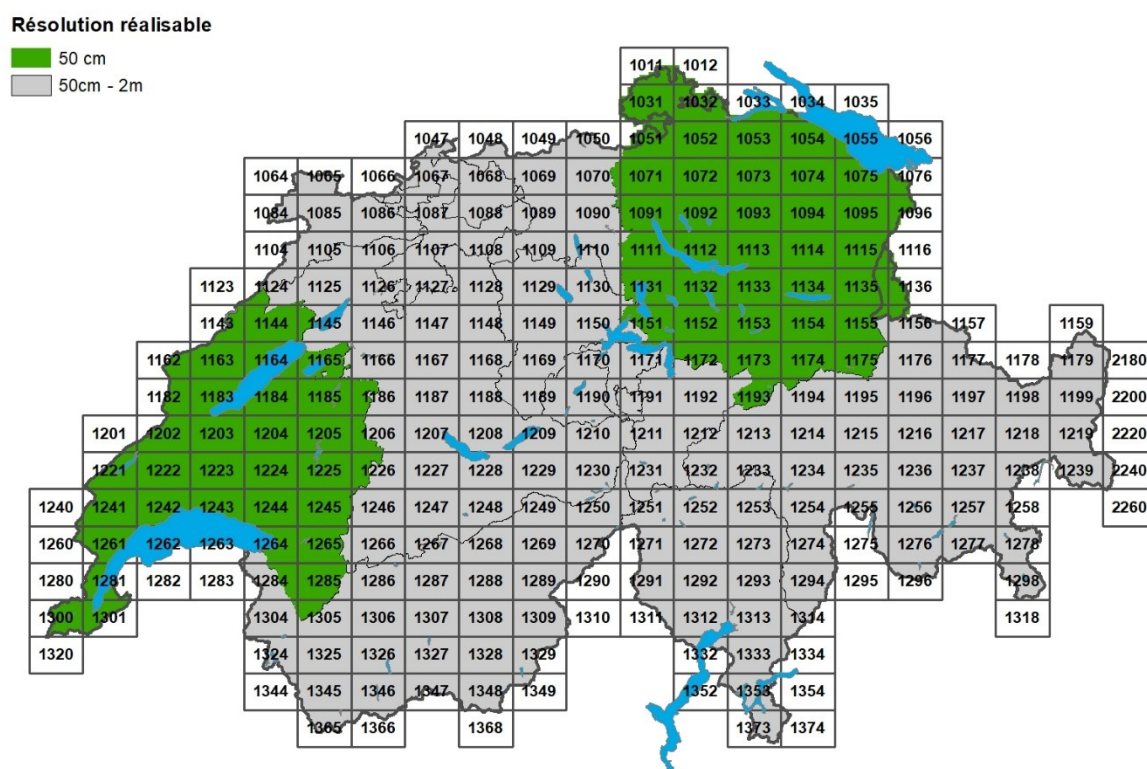
Figure 5: Résolution réalisable de swissALTI 3D en fonction de la densité de points des données de base
