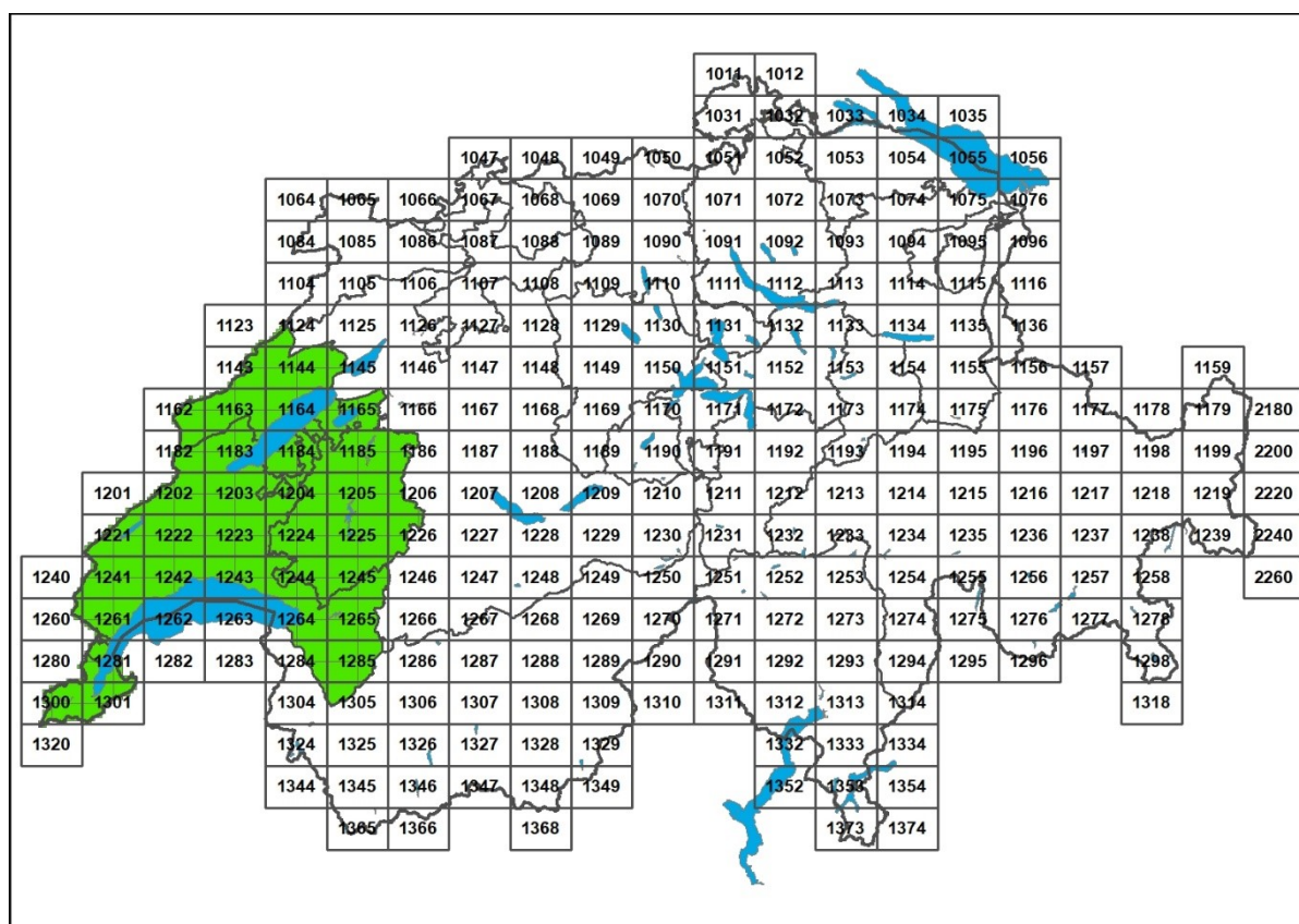
Figure 2: Régions actualisées pour la première publication de 2021
