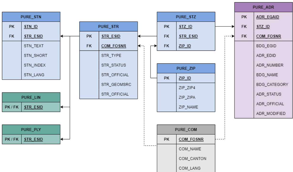
Abbildung 3-1: Relationales Datenmodell
