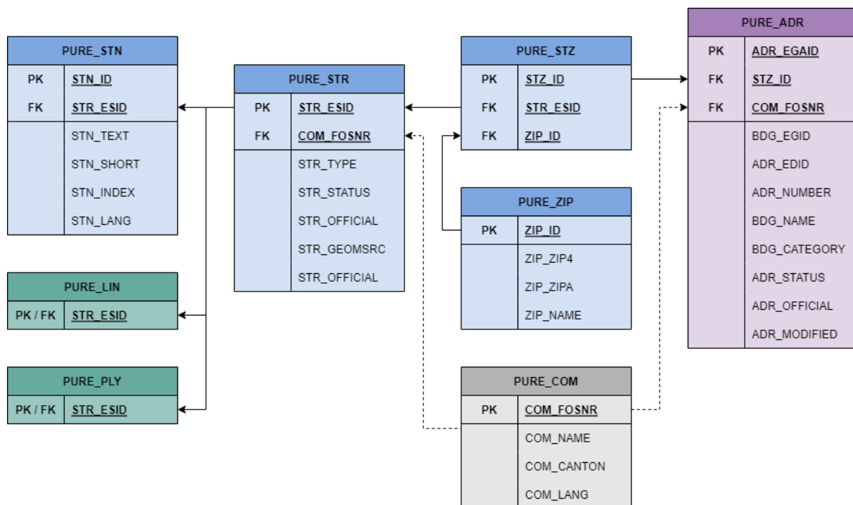
Figure 1: Modèle de données relationnel
